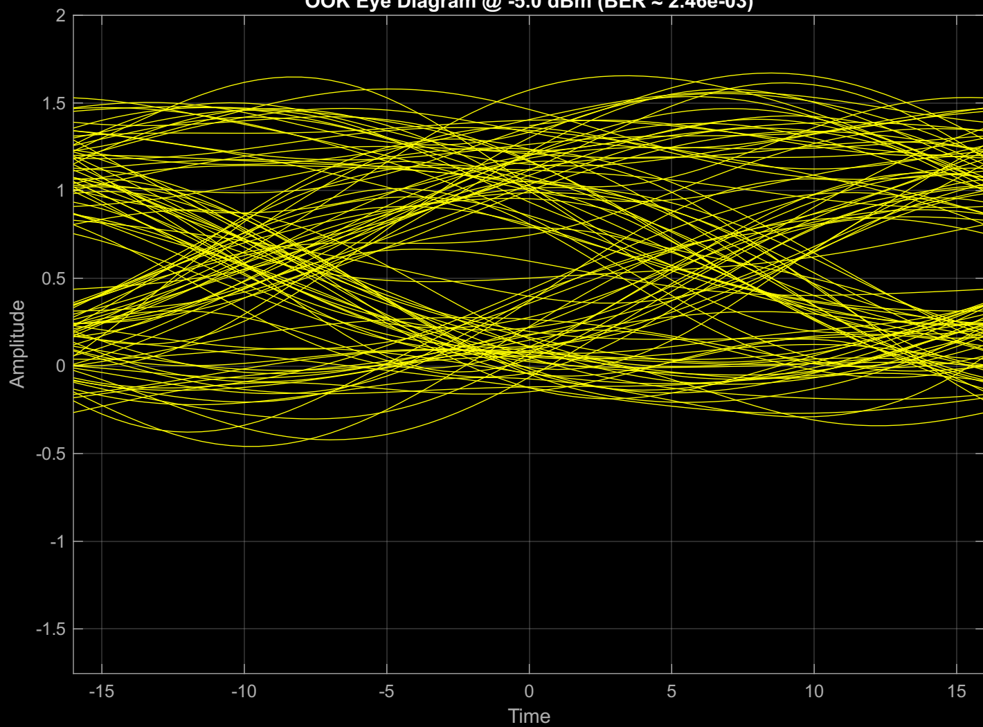
OOK Eye Diagram @ -5.0 dBm (BER \approx 2.46\text{e-}03 )
